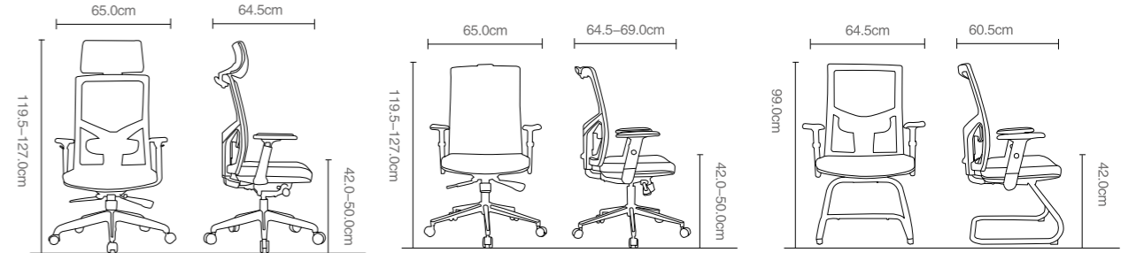
产品尺寸图 product dimensions
